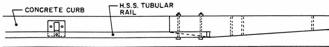
PLAN: BARRIER AND TERMINAL SECTION SCALE: N.T.S.
